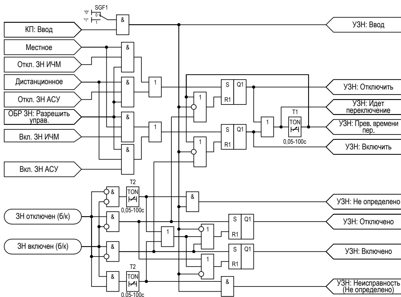
Рисунок 2.30 – Функциональная схема логики УЗН
